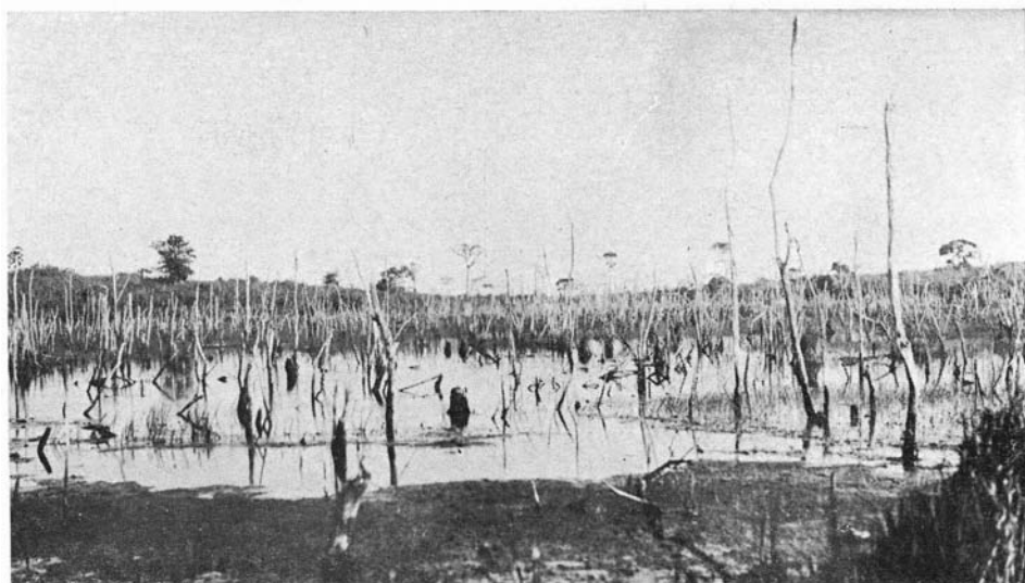
Fig. 23 — Uma lagoa salgada nos tabuleiros, ao norte de Campos
