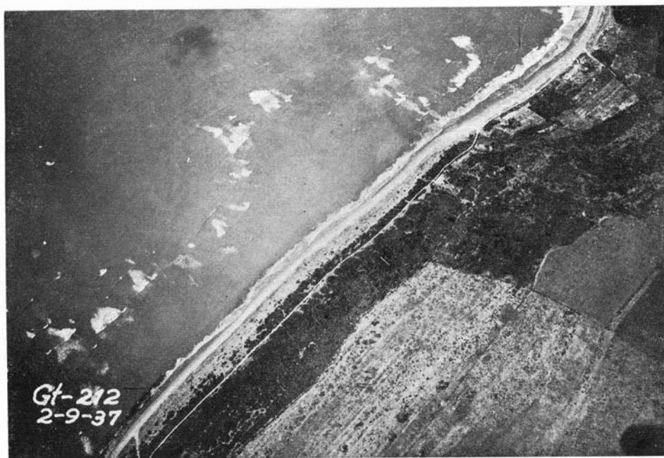
Fig. 38 — Restingas em Manguinhos, na costa norte fluminense. A arrebatção do mar 6 devida a afloramentos do arenito dos tabuleiros (AerofotoTe, Kafuri, do D.N.O.S.)
