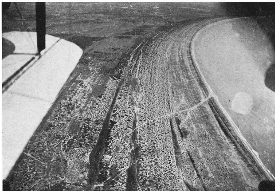
Fig. 29 — Planície de restingas mostrando o recuo do mar, ao norte da foz do Paraíba, na enseada de Gargáú
