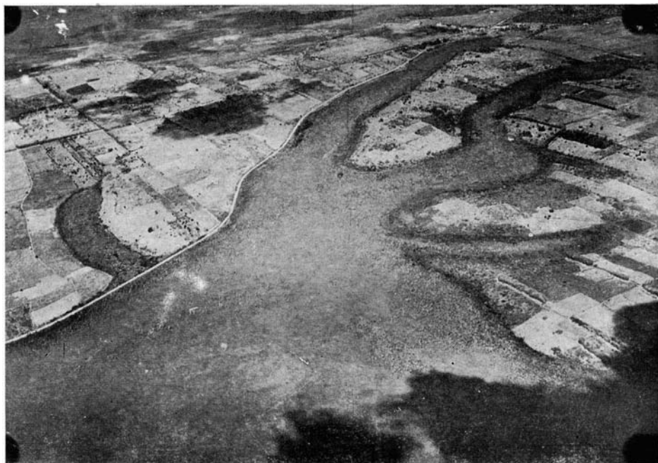
Fig. 13 — Região de tabuleiros ao norte de Dores de Macabú , que se vê ao alto (Aerofoto Te. Kafuri, do D.N.O.S.)
