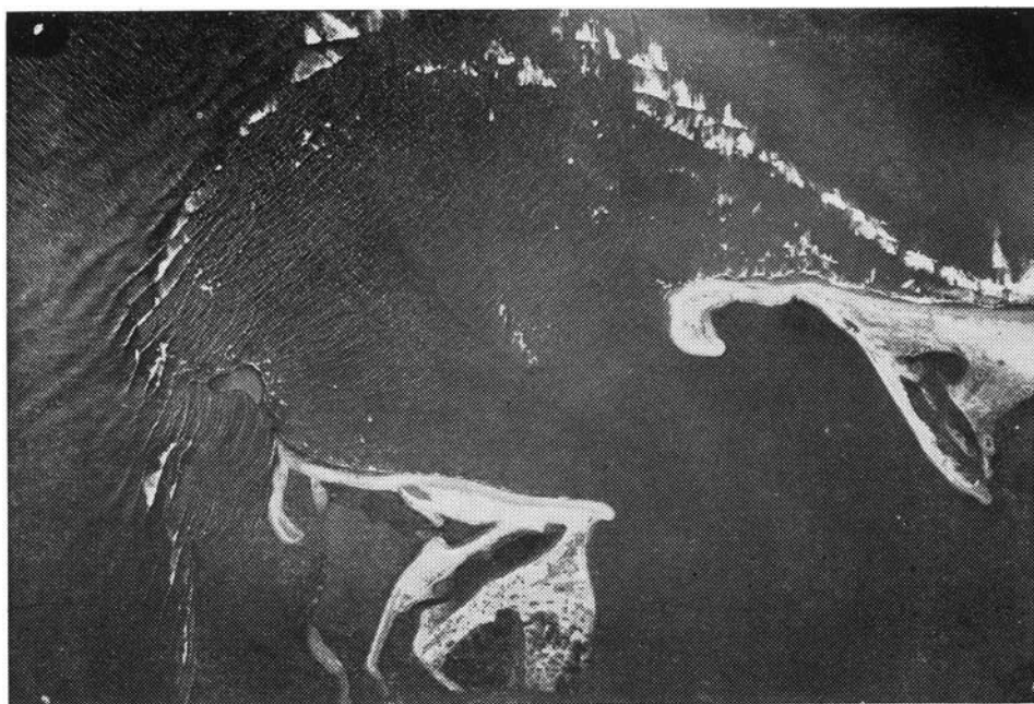
Fig. 128 — A foz do Paraíba em aerofoto vertical. Nota-se a mobilização da embo- cadura com o avanço das restingas para o norte.
