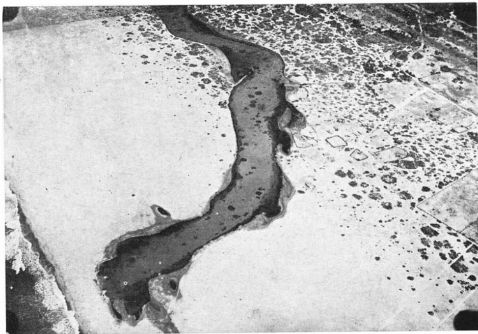
Fig. 31 — Foz da lagoa de Guruçal, fechada pelas areias (Aerofoto Te. Kafuri, do D.N.O.S.)
